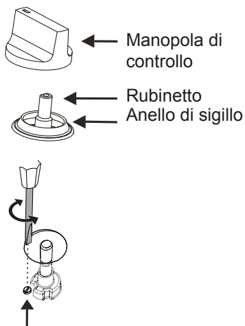
Vite di regolazione by-pass
